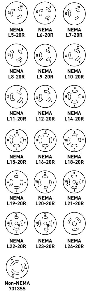
20A Connector
